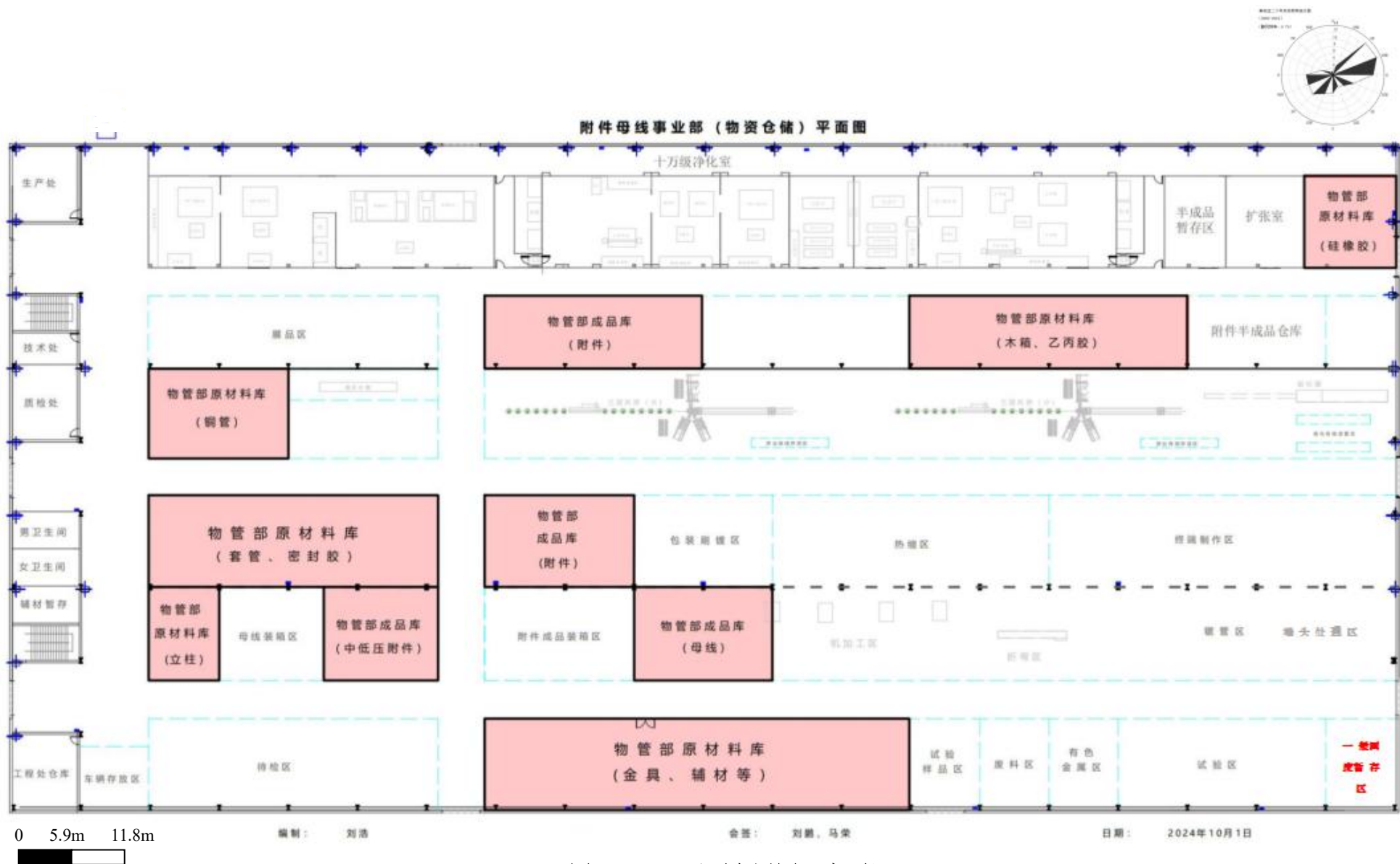
图 2.4-1b 平面布置图（本项目）
