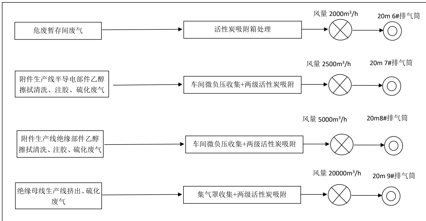
图 2.6-1 废气导排图
