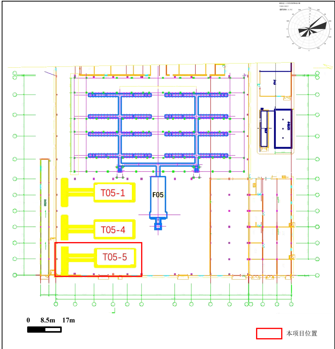
附图 3-1 项目 F05 车间内部平面布置图 (F05 车间)
